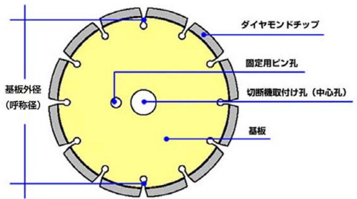
ブレード構成例
