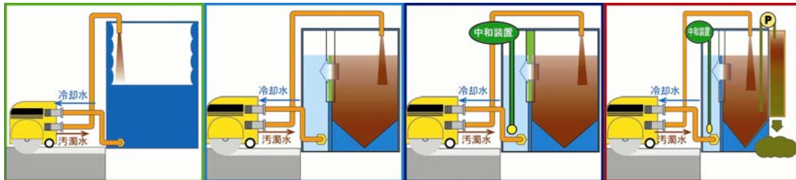
カッター汚水タンク 機能別処理範囲例
