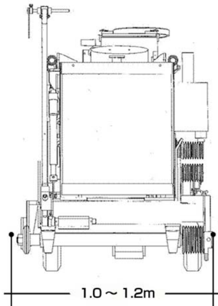
正面図
