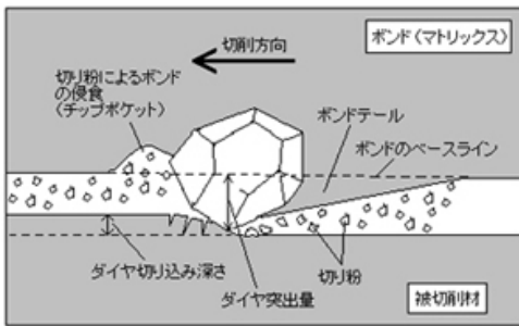
ダイヤモンドチップ磨耗工程
