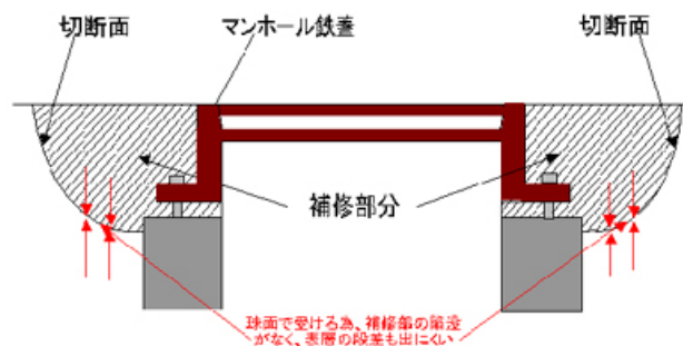
施工詳細断面図
